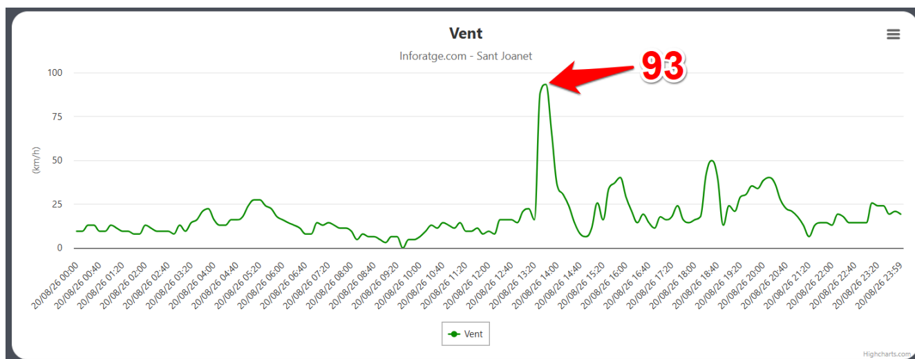
Ráfagas de viento registradas en SANT JOANET el 20/08/26 (en km/h) https://inforatge.com/meteo-santjoanet
